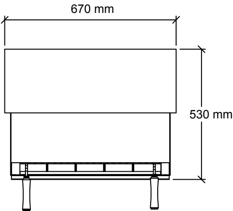
SCHÉMA DE PLAN PLAN DIAGRAM DIAGRAMA
