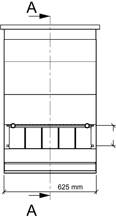
FAÇADE FRONT ELEVATION ELEVACIÓN FRONTAL
